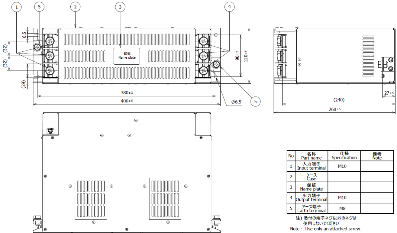
fig. 4 (200~300A)
